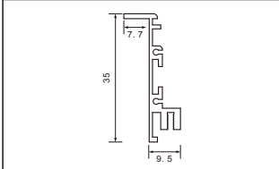
型号：35A折弯/73页
