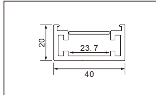
型号：4020M地踩折弯/78页
