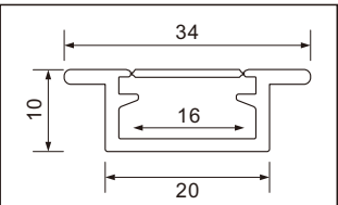
型号：2010A折弯/71页
