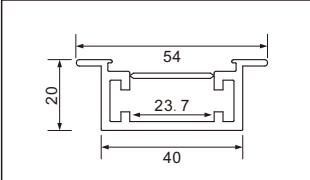
型号：4020A折弯/72页
