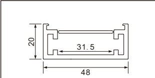
型号：4820M折弯/73页
