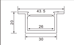
型号：3020A折弯/72页
