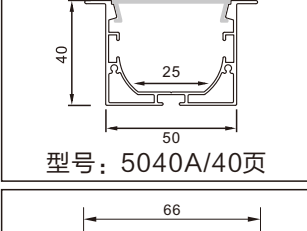
型号：5035A厚款/40页
