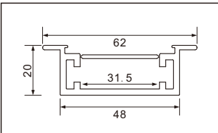
型号：4820A折弯/73页
