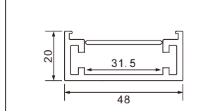
型号：4820M地踩折弯/78页
