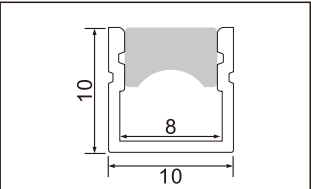
型号：1010M折弯/71页
