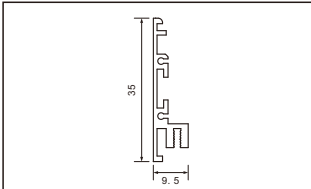
型号：35M折弯/73页
