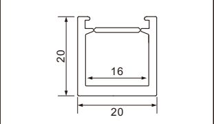
型号：2020M折弯/72页
