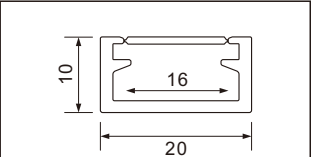
型号：2010M折弯/71页
