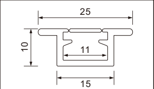
型号：1510A折弯/71页
