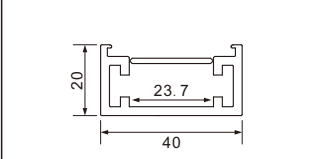
型号：4020M折弯/72页
