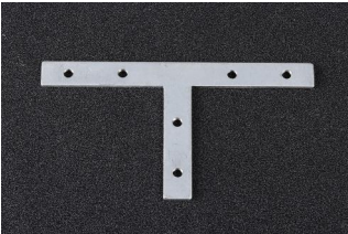
T字连接片 100mm*10mm*2mm 内六角M4螺丝
