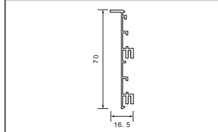
型号：70A折弯/76页
