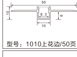
型号：1010单花边/50页
