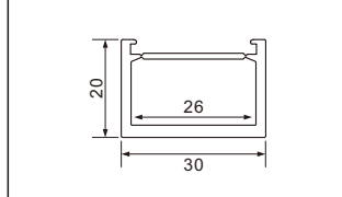
型号：3020M地踩折弯/78页
