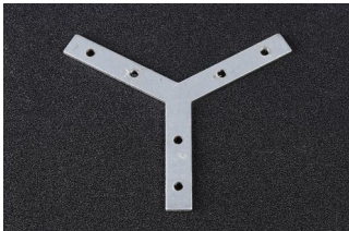
Y字连接片 100mm*10mm*2mm 内六角M4螺丝
