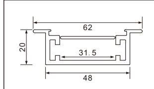
型号：4820A地踩折弯/78页
