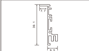
型号：40A折弯/74页
