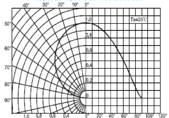
发光角度图 (极坐标)
