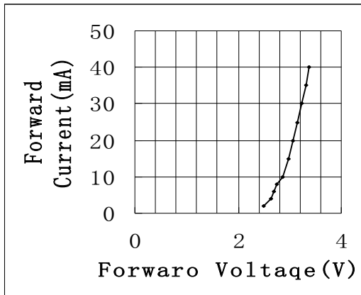
电压与电流关系曲线图
