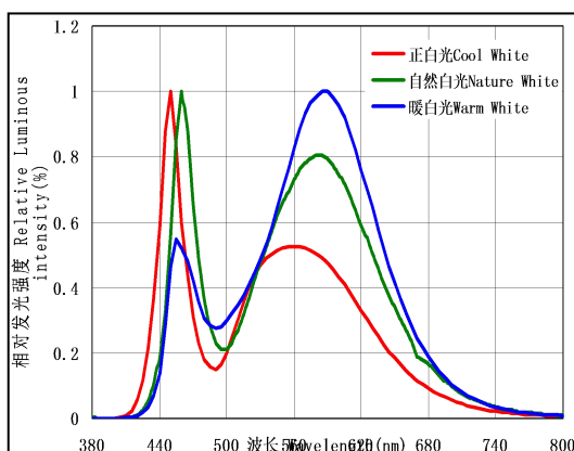
光谱特性图
